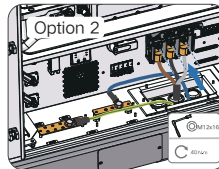
7-2 AC and equipotential bonding scheme 2
