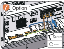
7-1 AC and equipotential bonding scheme 1
